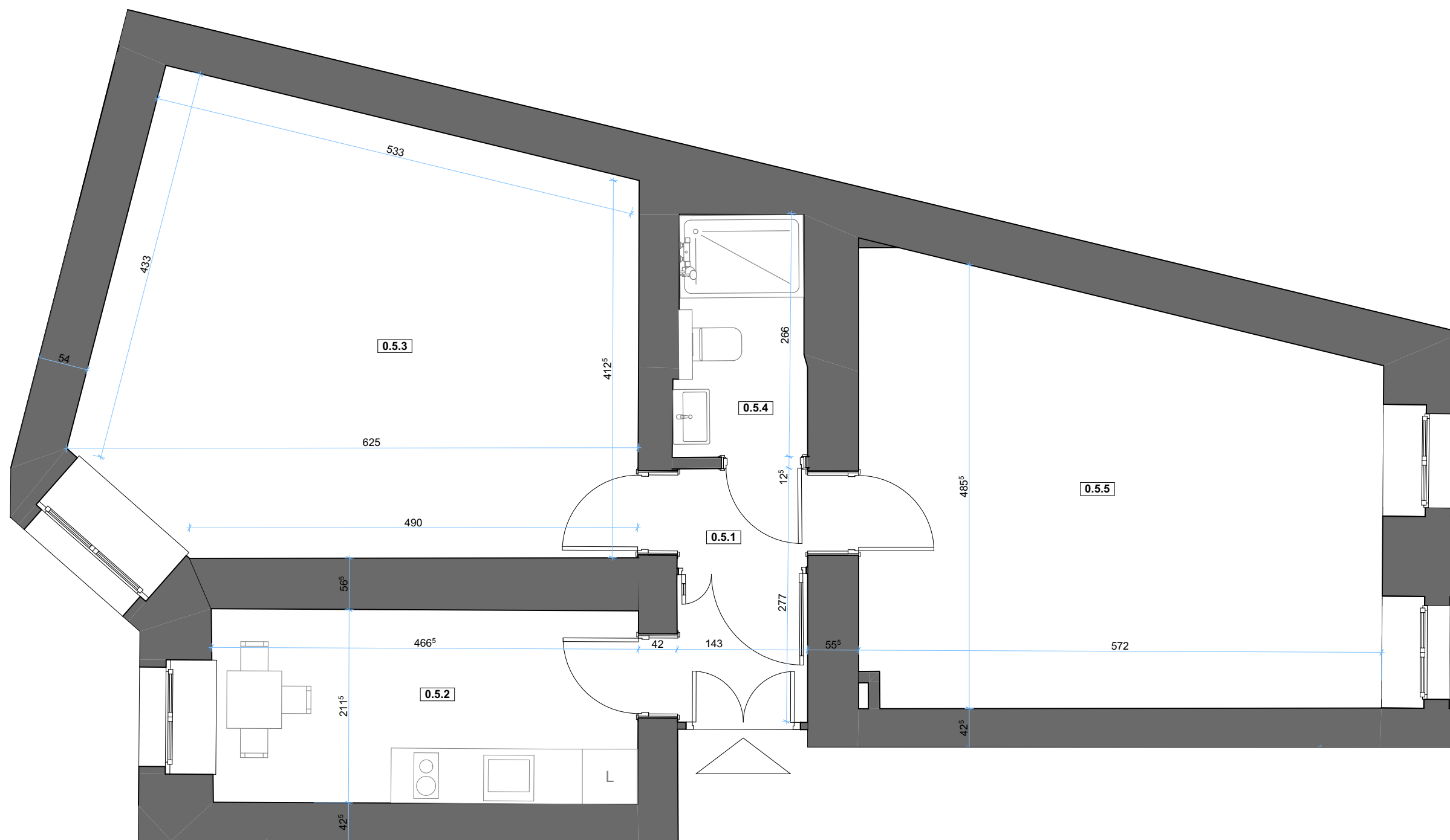
PLAN SYTUACYJNY, SKALA 1:50
