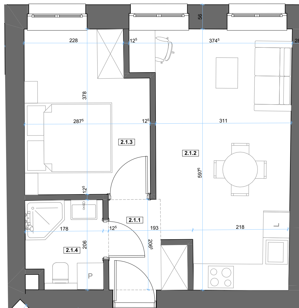
PLAN SYTUACYJNY, SKALA 1:50
