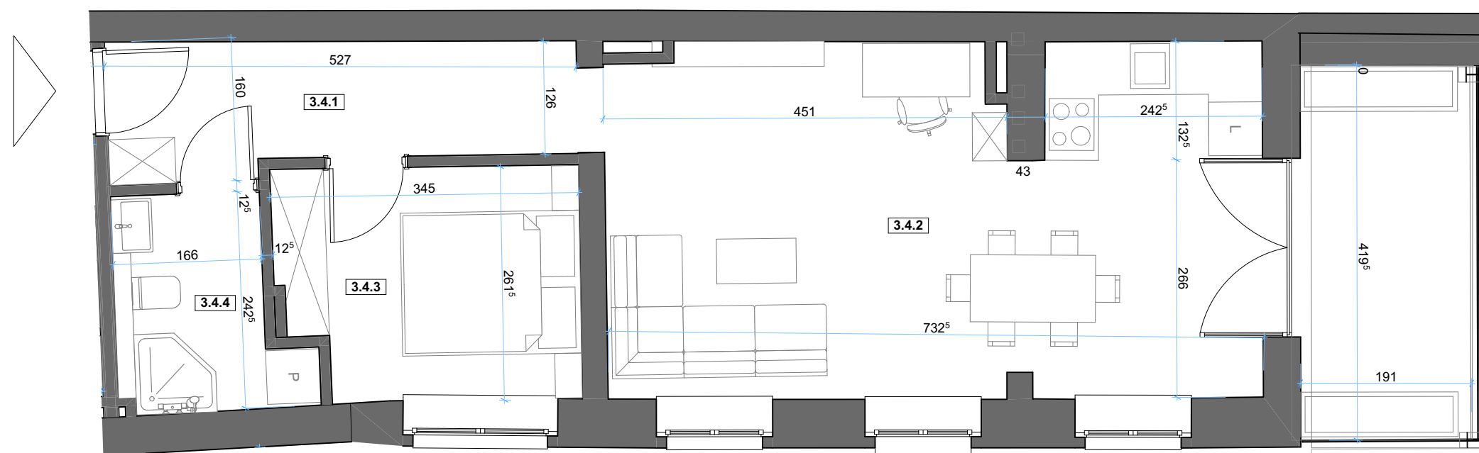
PLAN SYTUACYJNY, SKALA 1:60
