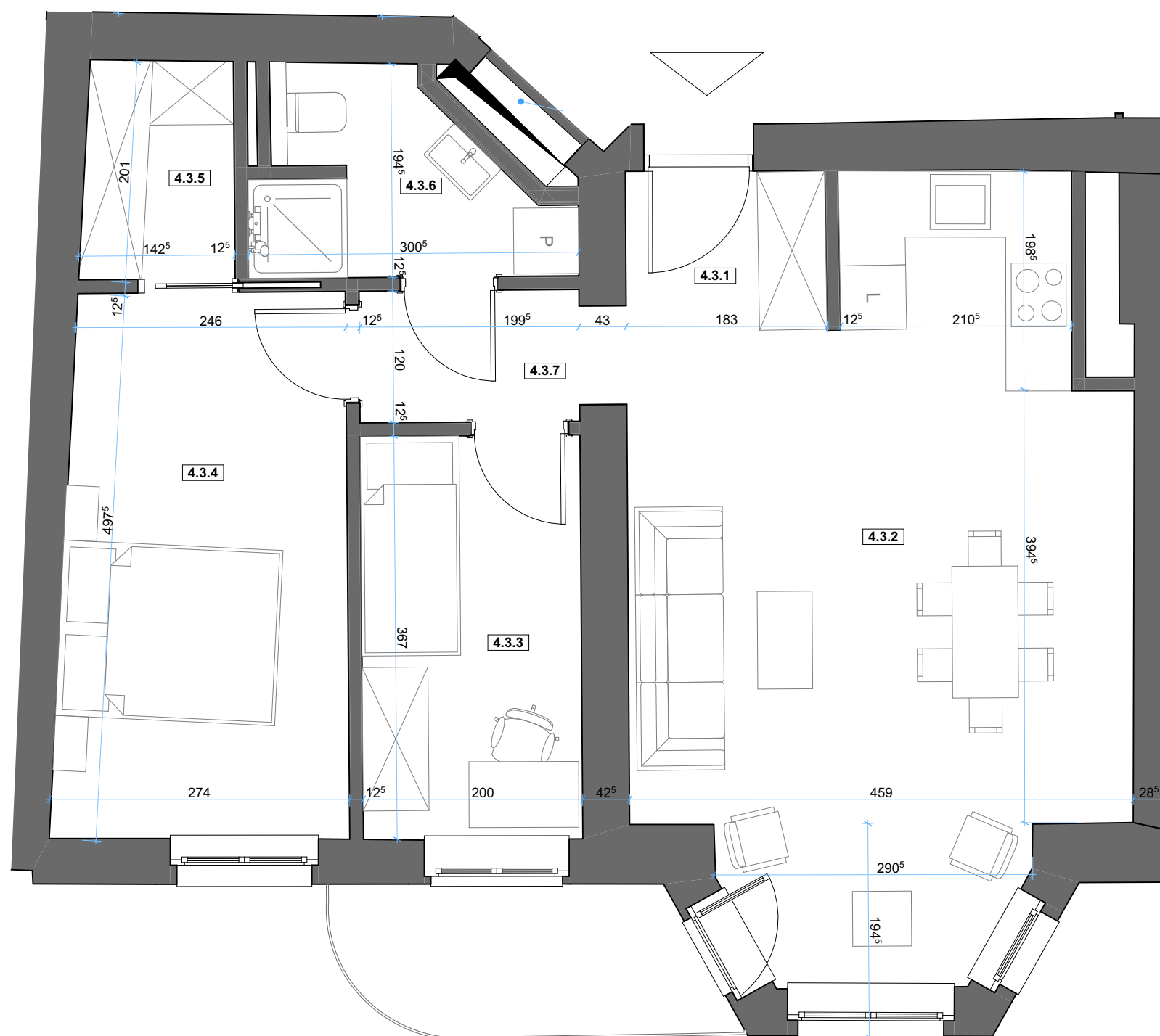
PLAN SYTUACYJNY, SKALA 1:50
