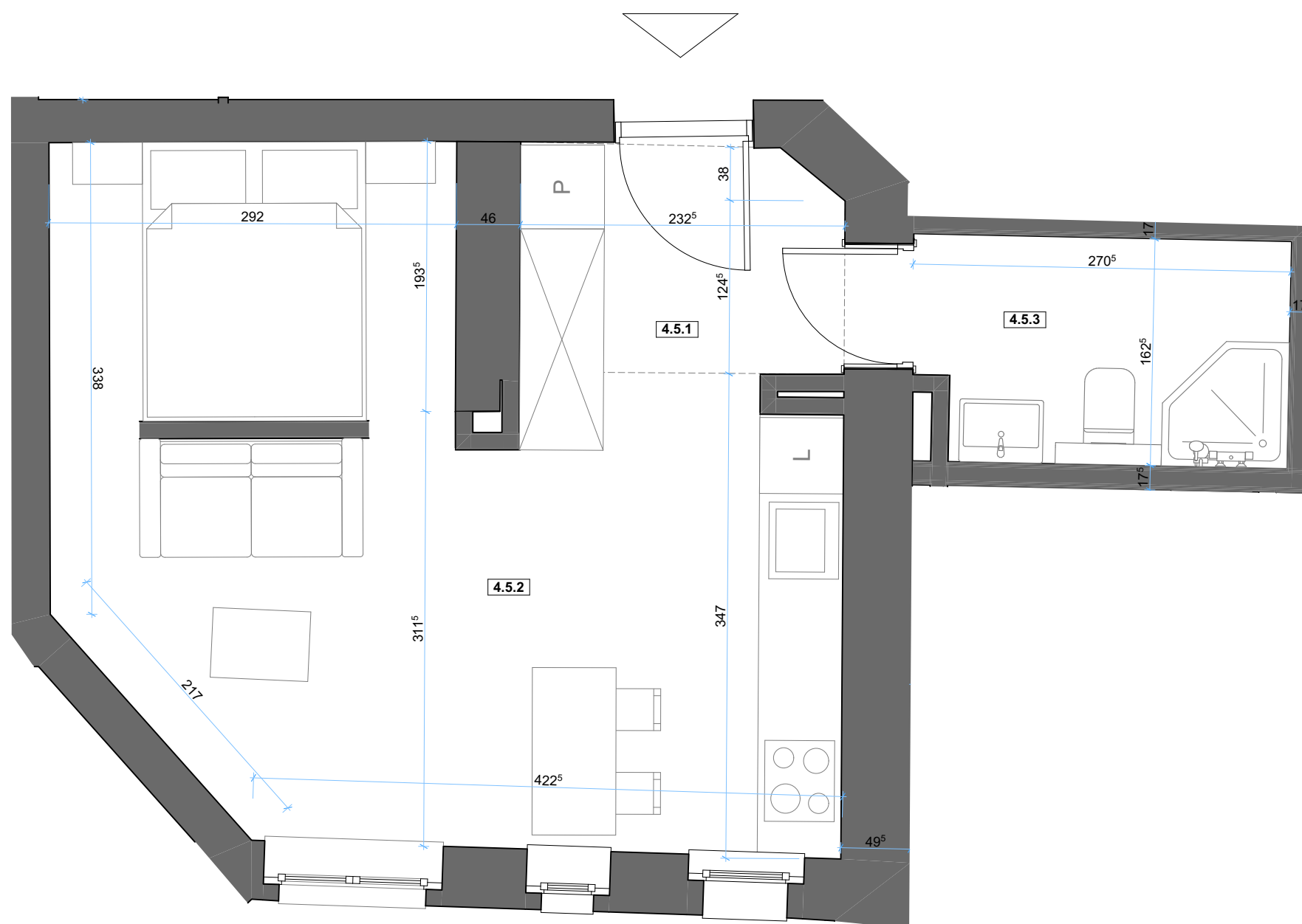
PLAN SYTUACYJNY, SKALA 1:40
