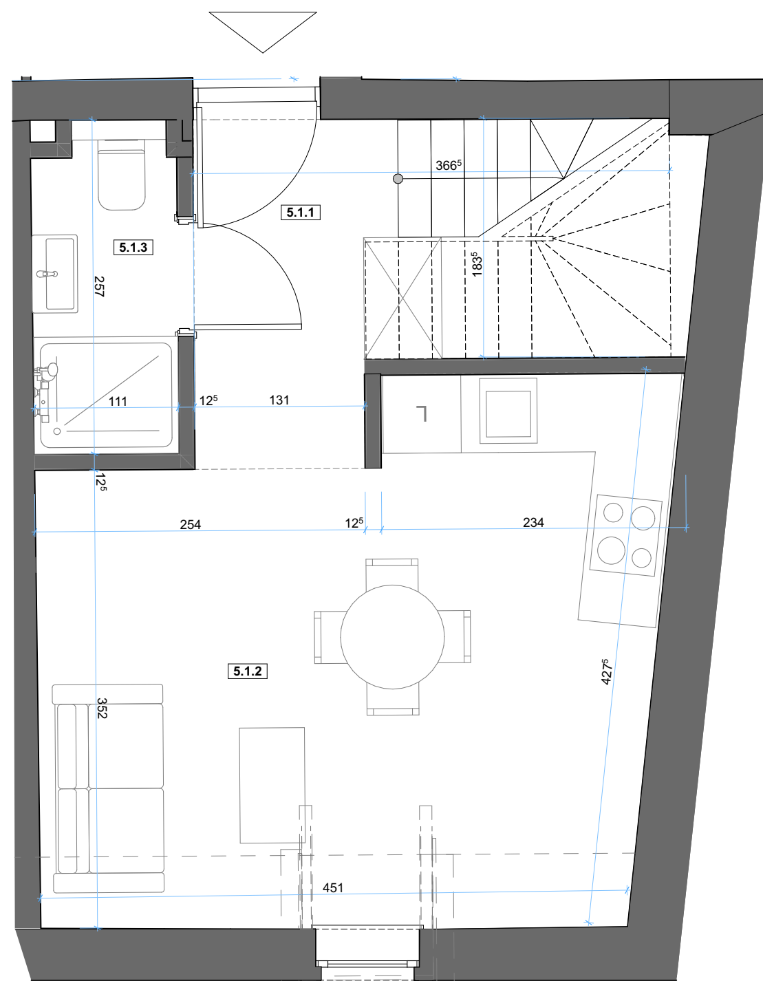
PLAN SYTUACYJNY, SKALA 1:40
