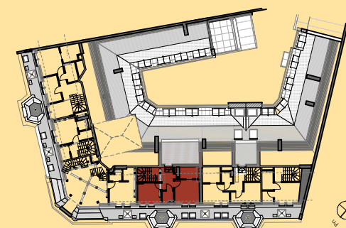
USYTUOWANIE LOKALU PIĘTRO +6
